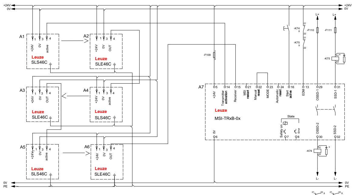
Bild 7.3: Sicherheits-Schaltgerät MSI-TRxB-xx mit 3x Typ 2 Einstrahl-Sicherheits-Lichtschranke SLS 46C in Reihe, Anlauf-/Wiederanlaufsperr (RES) und externer Schützkontrolle (EDM).
