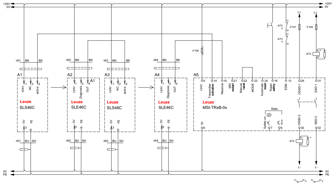
Bild 7.2: Sicherheits-Schaltgerät MSI-TRxB-xx mit 2x Typ 2 Einstrahl-Sicherheits-Lichtschranke SLS 46C in Reihe, Anlauf-/Wiederanlaufsperr (RES) und externer Schützkontrolle (EDM).
