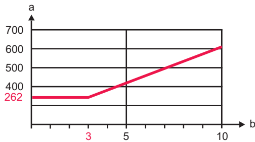
Bild 6.2: Mindestabstand zu reflektierenden Flächen je nach Schutzfeldbreite
