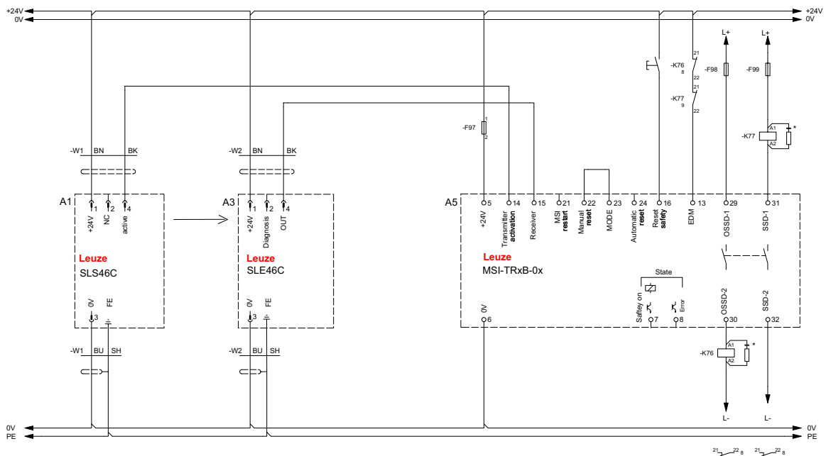
Bild 7.1: Sicherheits-Schaltgerät MSI-TRxB-xx mit Typ 2 Einstrahl-Sicherheits-Lichtschranke SLS 46C, Anlauf-/Wiederanlaufsperr (RES) und externer Schützkontrolle (EDM).
